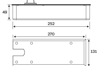
Dimension (mm.)
