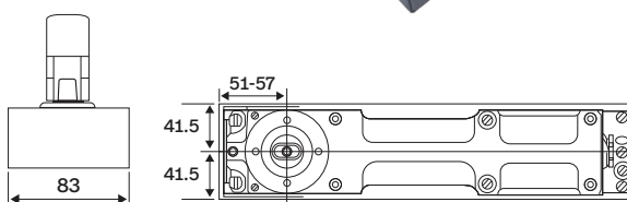
Dimension (mm.)
