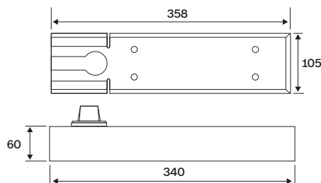
Dimension (mm.)
